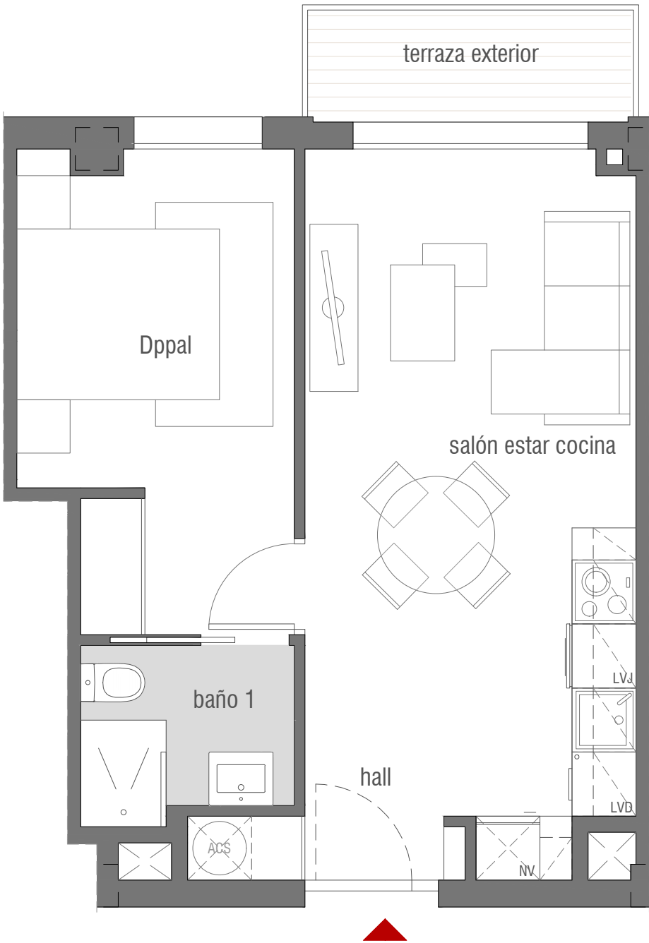
PLANTA SEGUNDA
