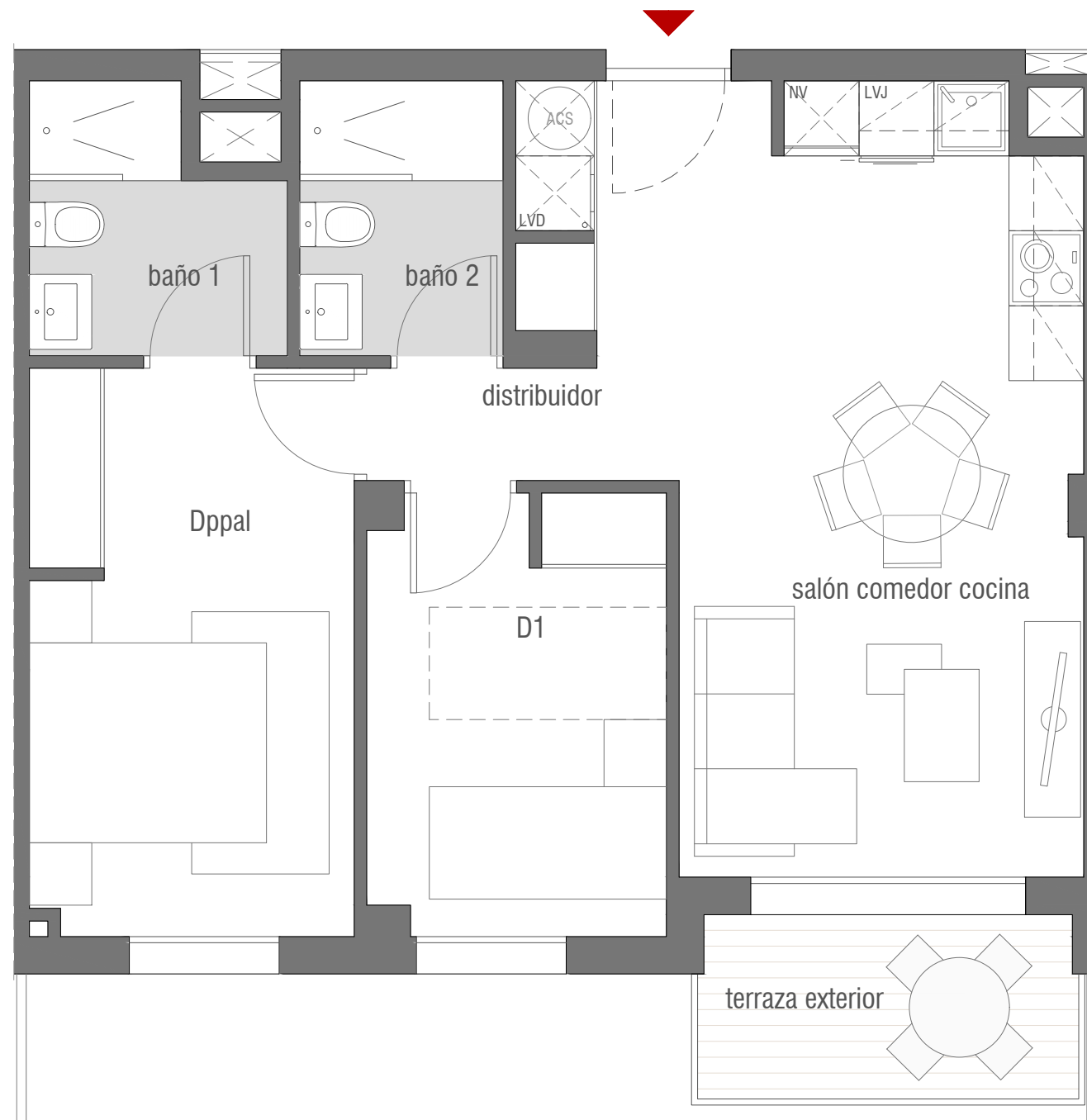
PLANTA PRIMERA
